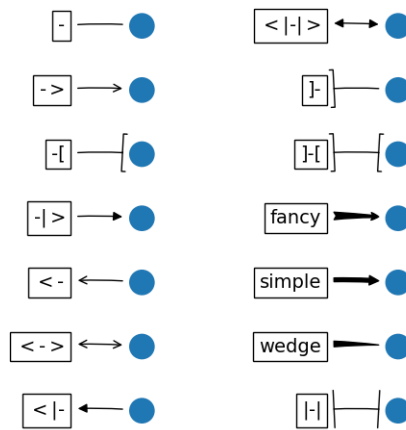
Fig. 30: Fancyarrow Demo
