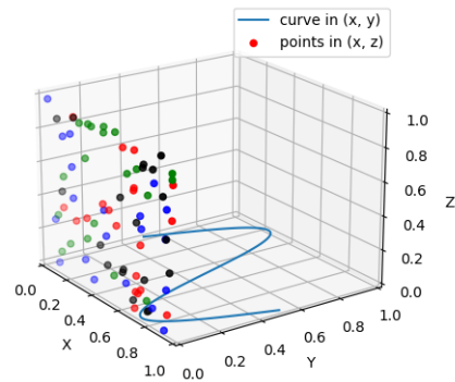
Fig. 86: 2dcollections3d
