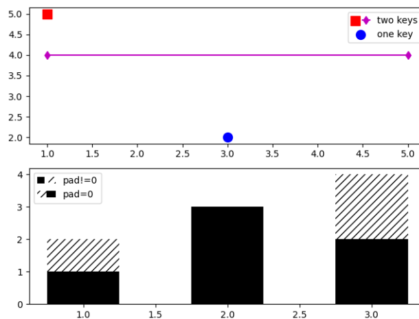
Fig. 22: Legend Demo4
