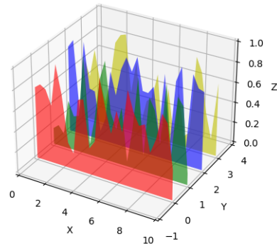
Fig. 83: Polys3d
