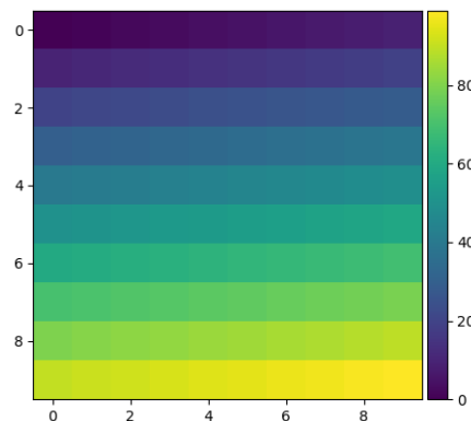
Fig. 51: Simple Colorbar
