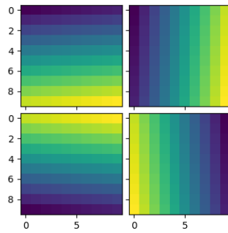
Fig. 48: Simple Axesgrid
