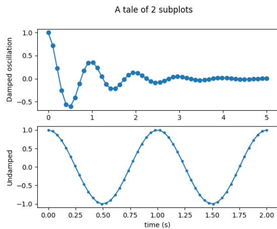
Fig. 2: Subplot
