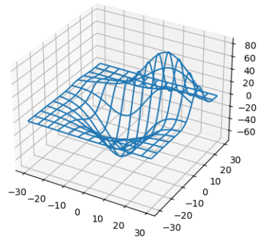
Fig. 78: Wire3d
