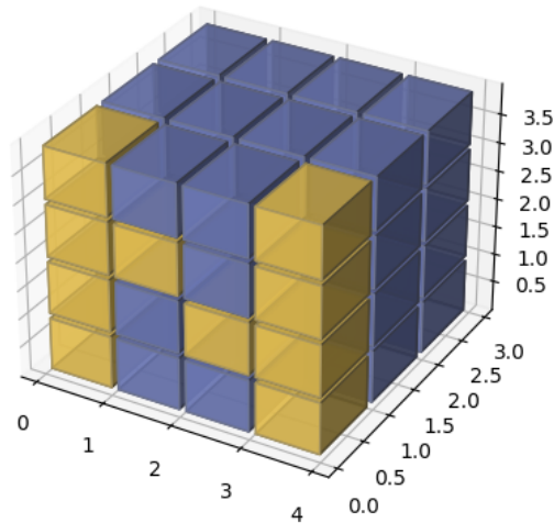
Fig. 3: Voxel Demo
