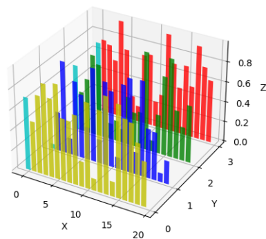
Fig. 84: Bars3d
