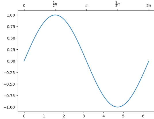
Fig. 54: Simple Axisline4
