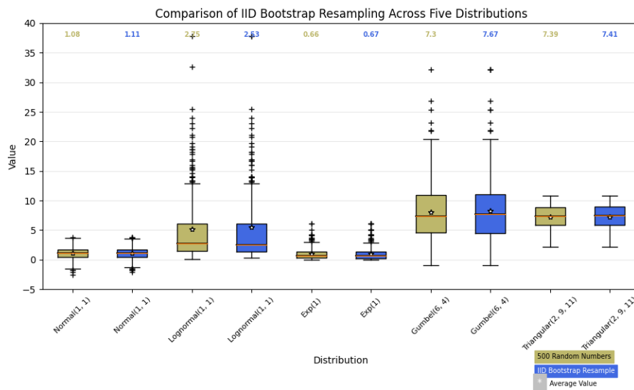
Fig. 17: Boxplot Demo3
