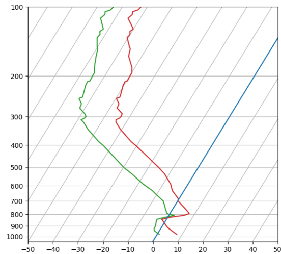
Fig. 8: Skewt
