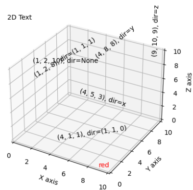
Fig. 87: Text3d
